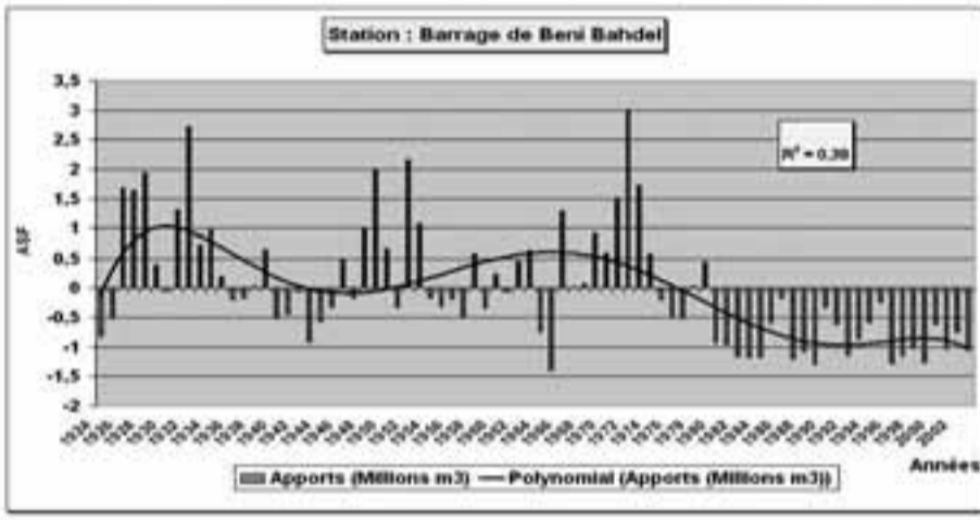
Fig. 28. Apports au barrage de Beni Bahdel (1924-2003)
