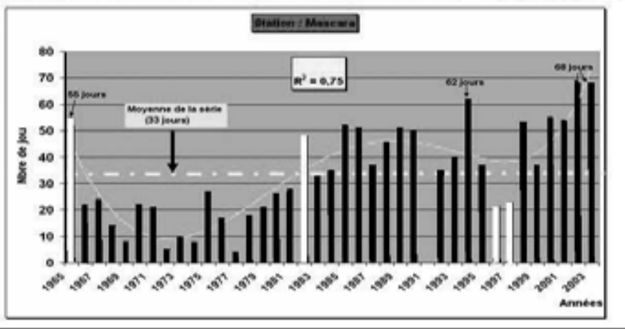
Fig.20: Nombre de jours de température maximale supérieure à 35°C
